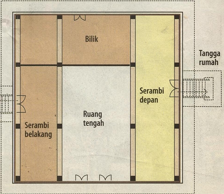
■ PELAN lantai rumah Kutai
