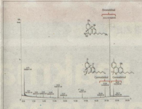
KROMATOGRAM daripada ujian makmal Eseri membuktikan terdapat unsur ganja semula jadi (kanabidiol dan kanabinol) dan ganja sintetik (dronabinol) dalam sampel cecair perisa vape.
